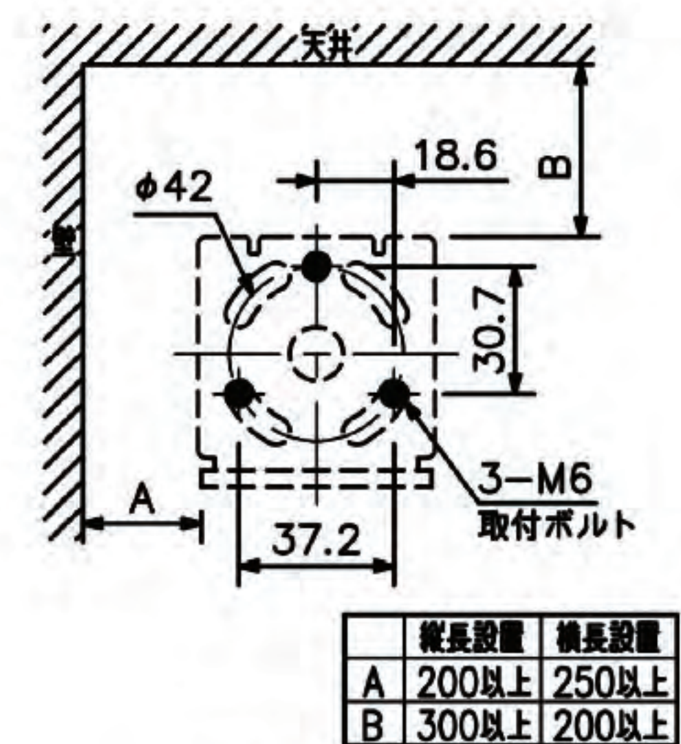
壁取付寸法 (ベース金具 (付属)) (縮尺: 1/3)
